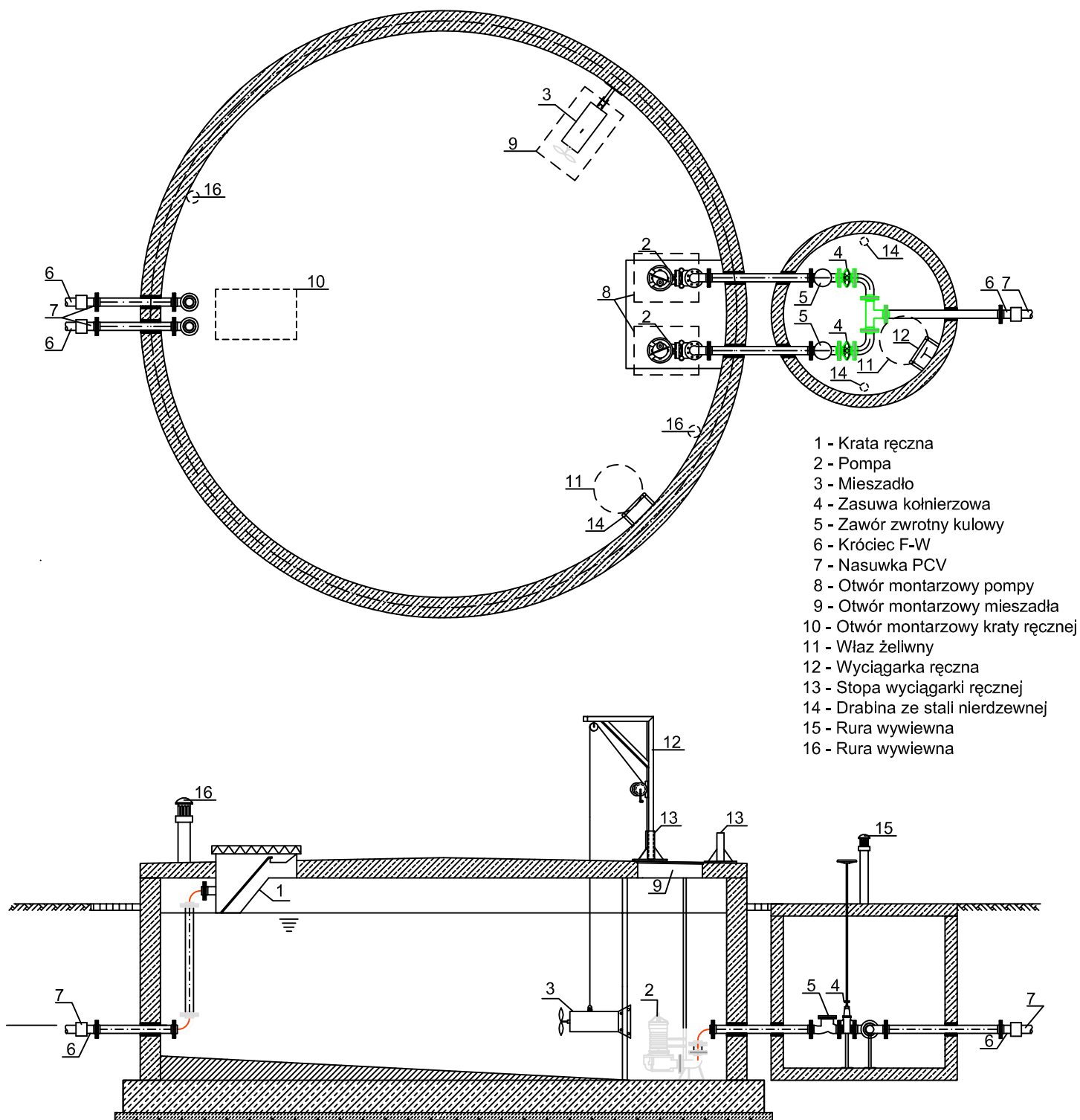
PRZEKRÓJ A-A
